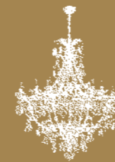
6469/12 V1165 Ø120 H130 12 E14 MAX 46W
