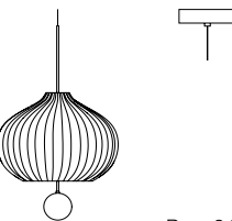
Lilli Ø 32 x H 52 Canopy Ø 12,5 x H 3
