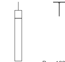
Minimal Ø 3,5 x H 25,5 Canopy Ø 6 x H 0,2
