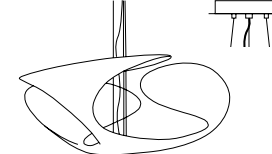
Clover Ø 70 x H 25 Canopy L 19,5 x W 19,5 x H 3
